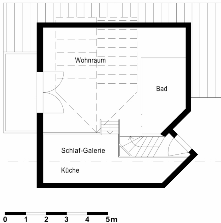
Grundriss
